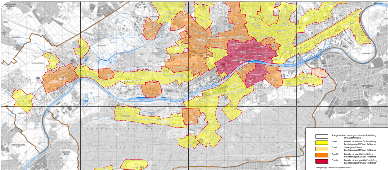
Abbildung 17: Zonen der Erschließungsqualität im Öffentlichen Nahverkehr (ÖV) und der Einschränkung der Kfz-Stellplätze in der Stellplatzsatzung Frankfurt am Main.
