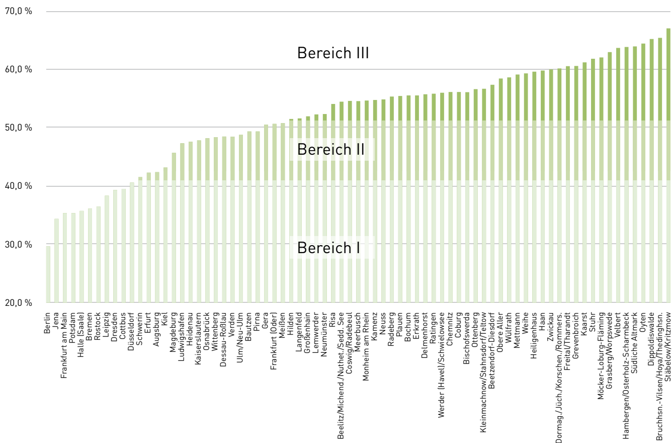
Abbildung 13: MIV-Anteil an allen Wegen der Einwohner (2013); Datenquelle: TU Dresden, Fakultät Verkehrswissenschaften „Friedrich List“, Institut für Verkehrsplanung und Straßenverkehr: Sonderauswertung zum Forschungsprojekt „Mobilität in Städten – SrV 2013“ – Städtevergleich. Dresden, März 2016.
